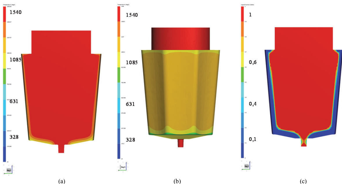
Obr. 4 Teplotní pole (°C) po odlití - po průřezu ingotu (a), povrch ingotu (b), podíl tekuté fáze po dokončení liti (c)
