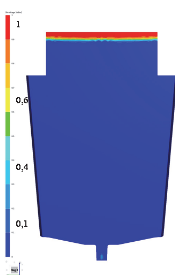
Obr. 6 Smrštění 1,6 t ingotu Obr. 6 Shrinkage of the 1.6 t ingot
