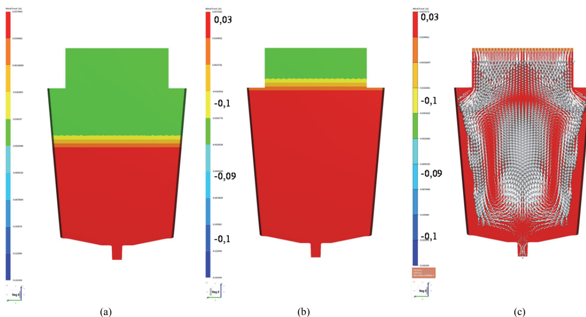
Obr. 3 Plnění kokily taveninou při 50 % (a), 90 % (b), vektorový tok taveniny při 99 % zaplnění (c)
