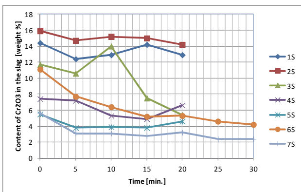
Obr. 10 Průběh obsahu Cr_2O_3 ve strusce u všech experimentů Fig. 10 Evolution of Cr_2O_3 content in the slag in all experiments
