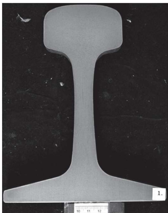
Obr. 1 Středová segregace ve stojině kolejnic Fig. 1 Central segregation in rail webs
