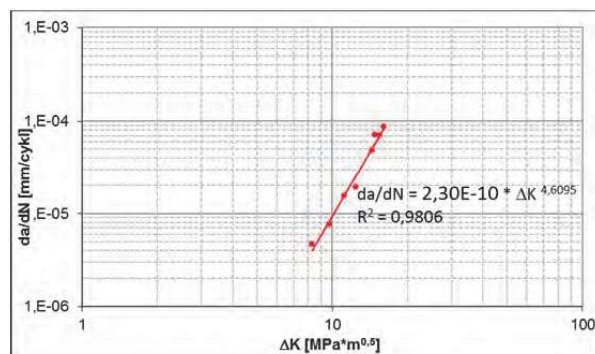
Obr. 4 Příklad stanovení závislosti rychlosti šíření únavové trhliny na rozkmitu faktoru intenzity napětí v oblasti Parisova vztahu na materiálu IH 350
