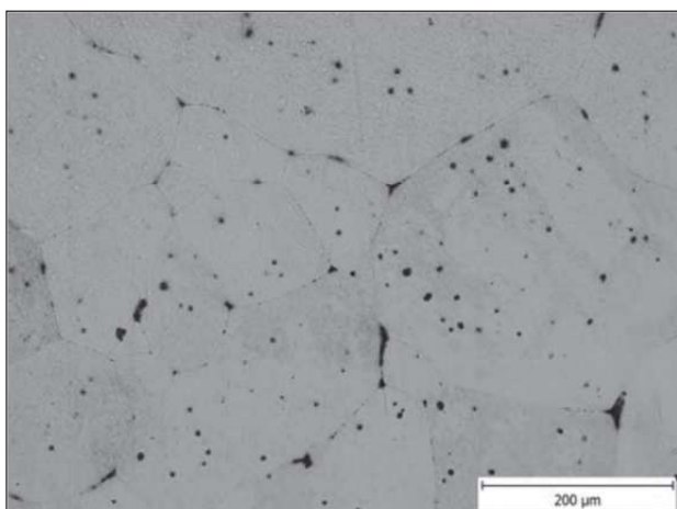
c) výchozí protvářěný strukturní stav, teplota ohřevu 1370 °C c) initial formed structural state, heating temperature of 1,370 °C
