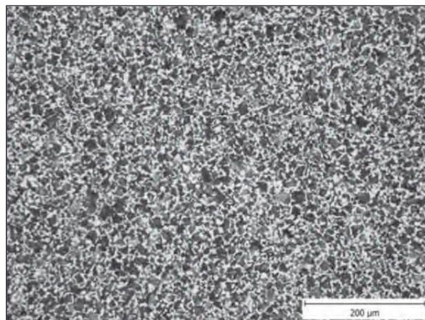
Obr. 1 Mikrostruktura za tepla válcovaných tyčí Fig. 1 Microstructure of the hot rolled bars
