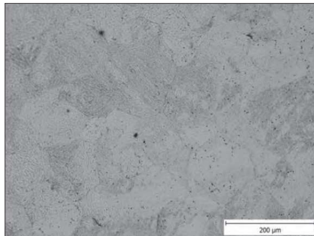
b) výchozí protvářěný strukturní stav, teplota ohřevu 1200 °C b) initial formed structural state, heating temperature of 1,200 °C
