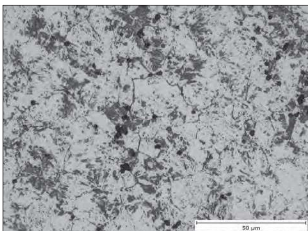
a) výchozí protvářěný strukturní stav, teplota ohřevu 900 °C a) initial formed structural state, heating temperature of 900 °C
