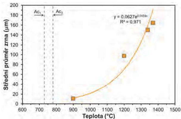
Obr. 4 Vliv teploty ohřevu na střední průměr zrna zkoumané oceli v protvářeném výchozím stavu
