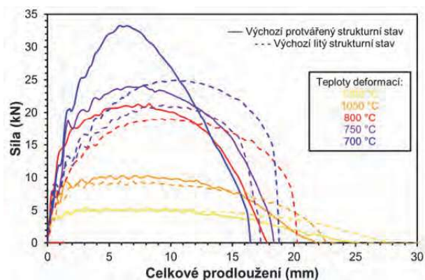
a) rychlost tažení 1000 \text{mm}\cdot\text{s}^{-1} a) tensile rate of 1,000 \text{mm}\cdot\text{s}^{-1}
