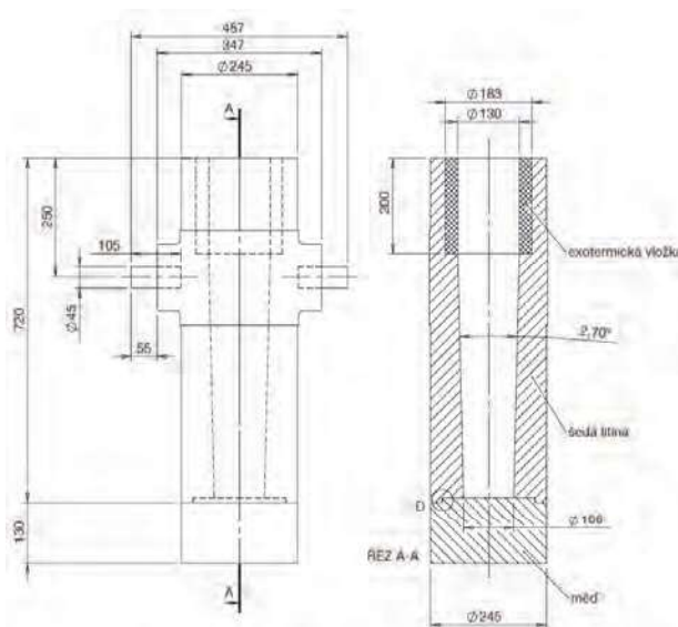
Obr. 5 Kokila pro odlévání experimentálních ingotů
