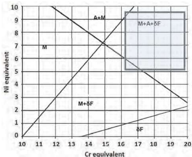
Obr. 3 Schneiderův diagram – vyznačena oblast rozpětí chemického složení oceli 14Ch17N2 dle GOST 5632
