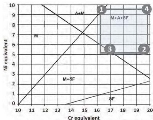
Obr. 4 Schneiderův diagram – pozice čtyř experimentálních taveb v oblasti rozpětí chemického složení oceli 14Ch17N2
