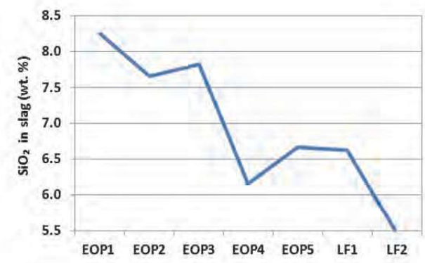
Fig. 12 The course of the content of SiO 2 in slag during X2CrNiMo13-4 steel production and processing Obr. 12 Průběh obsahu SiO 2 ve strusce během výroby a zpracování oceli X2CrNiMo13-4
